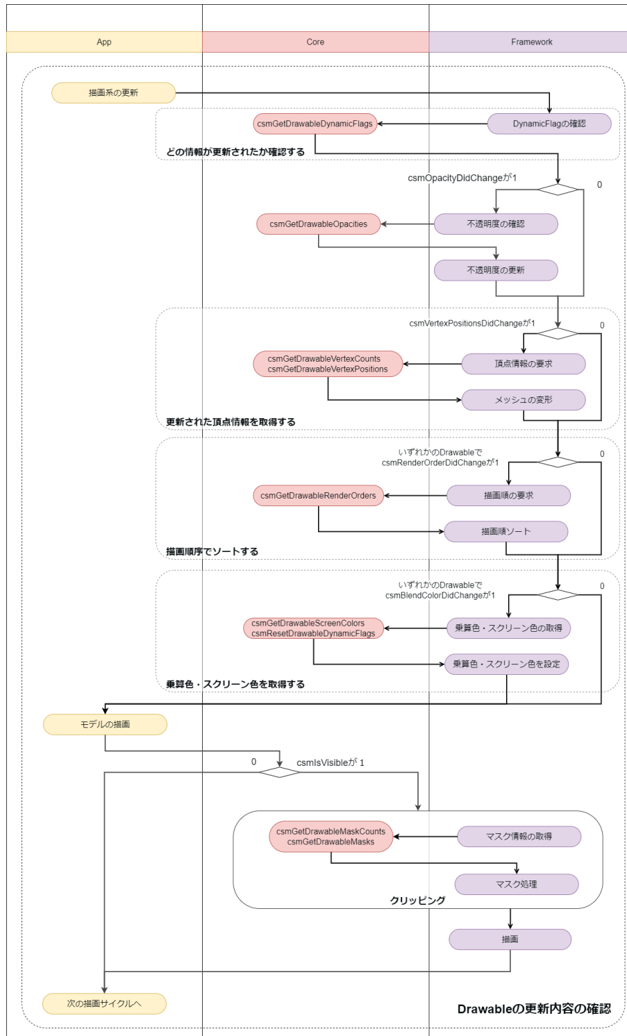
フラグの確認処理のフロー図
